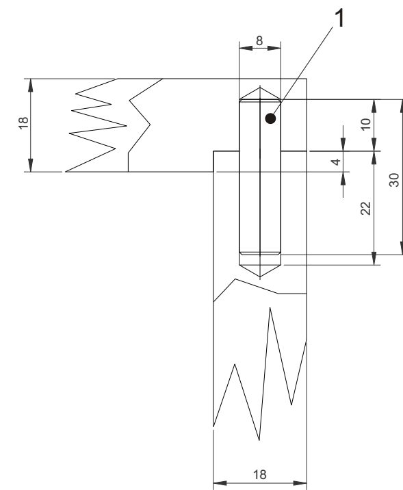
Einzelheit X M 1:1
